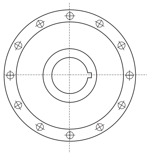
Agujero pasante o roscado
