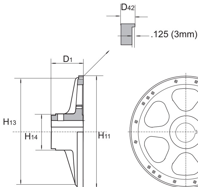
Porta Llanta ① tamaño 20 al 24
