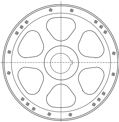
Tamaño 16 en adelante
