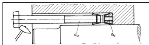
Figura 19: Atascamiento del cono frontal Si el contratrote frontal se atasca, extraiga los 3 tornillos cromatizados en zinc para liberar las roscas ( d_D ) del cono frontal. Inserte los tornillos o varillas roscadas correspondientes (ver herramientas de extracción) y pulse ligeramente hacia afuera para liberar el cono frontal. Las roscas extraíbles solo tienen de 3 a 5 filetes efectivos; no son adecuadas para realizar fuerza de extracción potente y solo deberán utilizarse para extraer el acople BLOKEAR 200 EN CASO DE ENGRANE .
